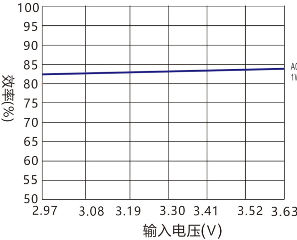
效率Vs输入电压 (满载)
