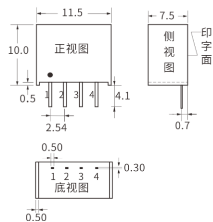
1)外观尺寸(单位: mm,公差: xx ±0.25)
