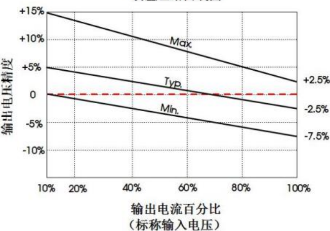
5VDC 输出 误差包络曲线图
