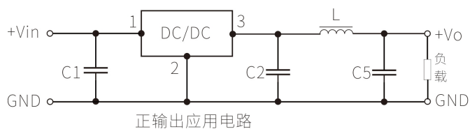
图3 ‘LC’ 滤波应用电路
