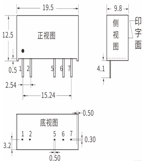
产品外观尺寸及引脚定义、建议印刷版图
