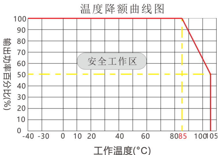
图 1 (温度降额曲线)
