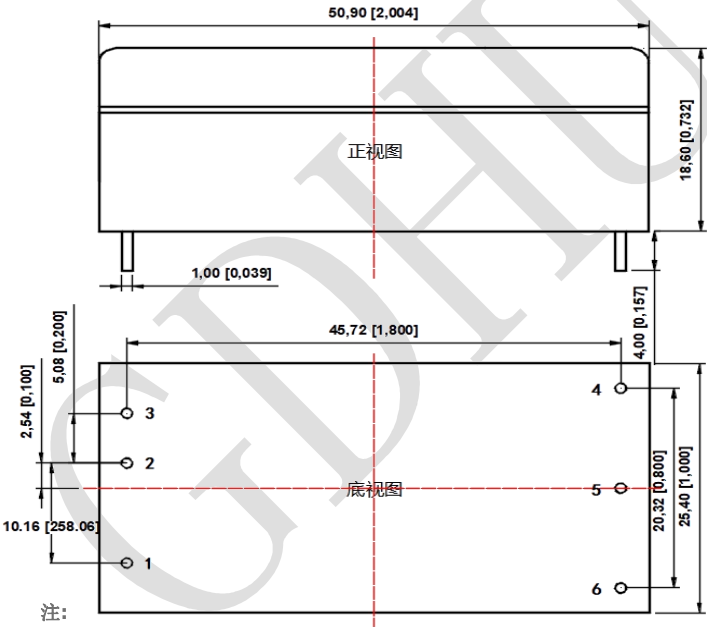
URBxxxxLD-60WHR3(加散热片)尺寸图
