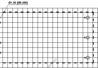
栅格距离尺寸为 2.54 x 2.54 mm
