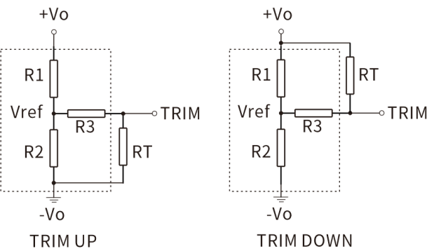
Trim 的使用电路(虚线框为产品内部)
